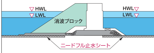
防波堤
