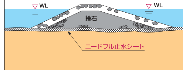
離岸堤
